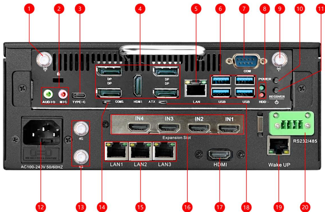
后面板
